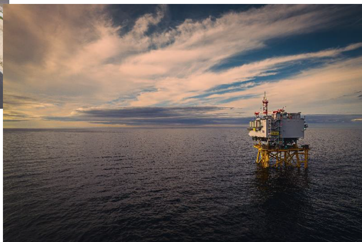
©Parc éolien en mer du Calvados
